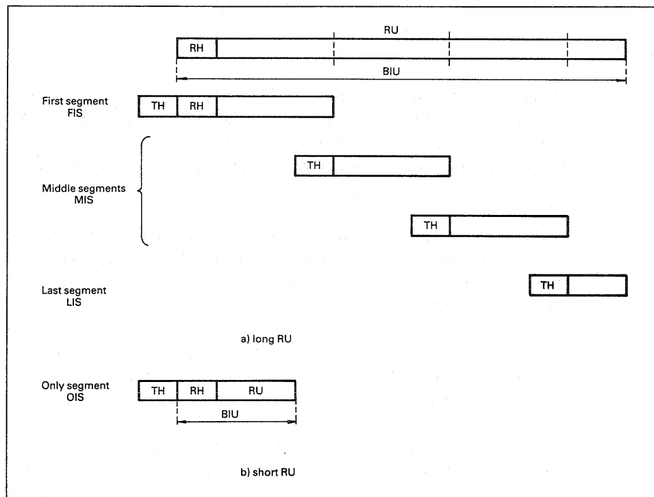
Fig. 4. Segmenting of RUs
